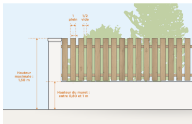
Mur bahut surmonté d'un dispositif à claire-voie
